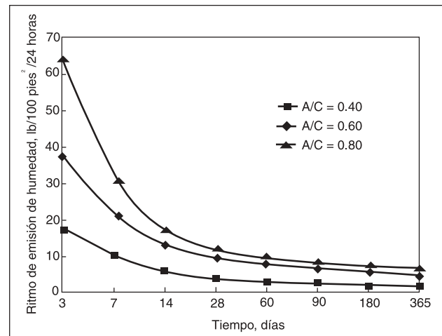
Figura 1. Tasas de secado de concretos ( hormigones ) sellados en el fondo (ref. 3)
